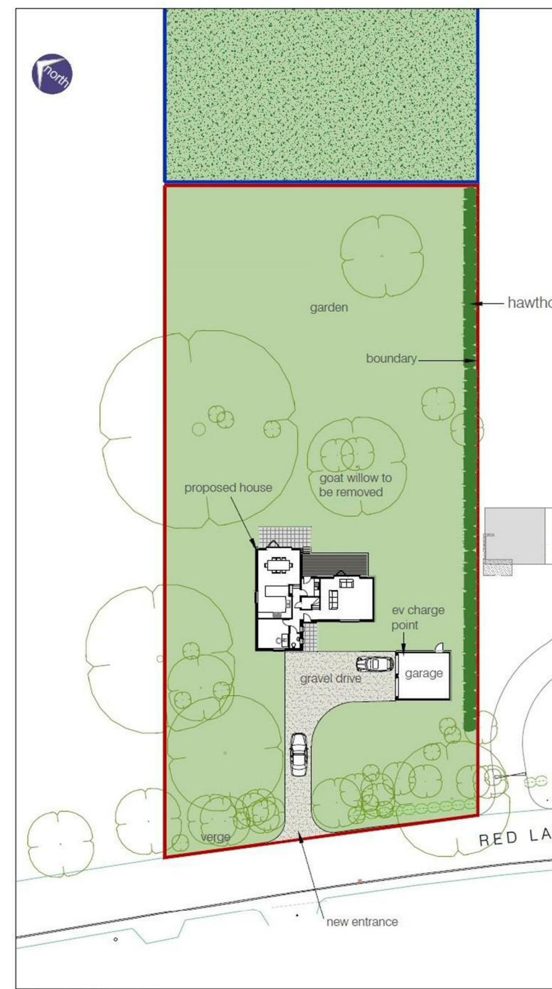
SITE PLAN 1:500
