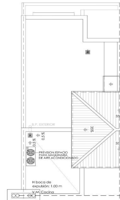
PLANTA DE CUBIERTA
