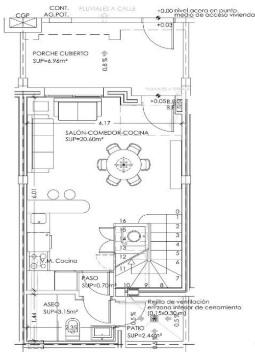
PLANTA BAJA
