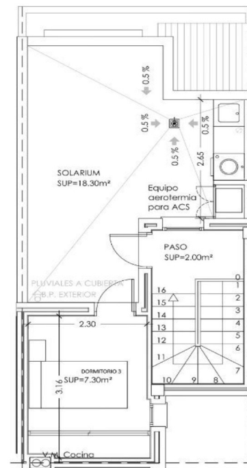
PLANTA TRASTERO
