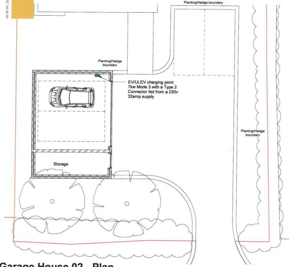
Garage House 02 - Plan 1 : 100
