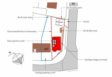
9 SITE PLAN 1 : 500
