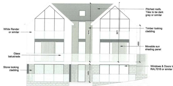
West - House 01 1 : 100
