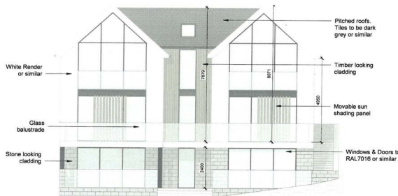
West - House 01 1 : 100
