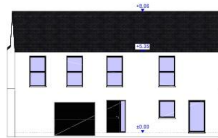
Façade sud-ouest
