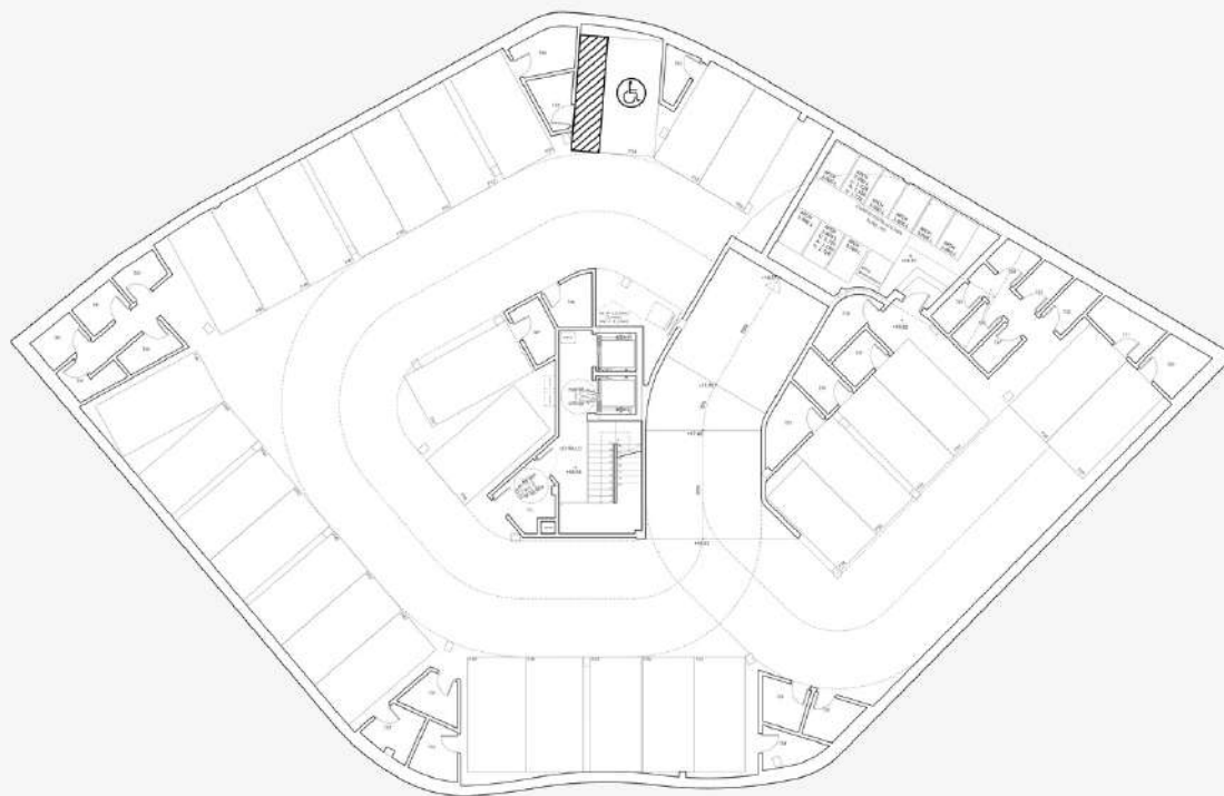
LEVEL - 1 / NIVEL -1
