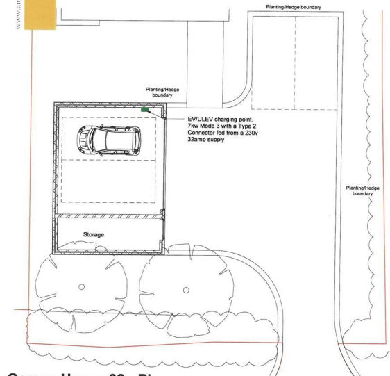
Garage House 02 - Plan 1 : 100
