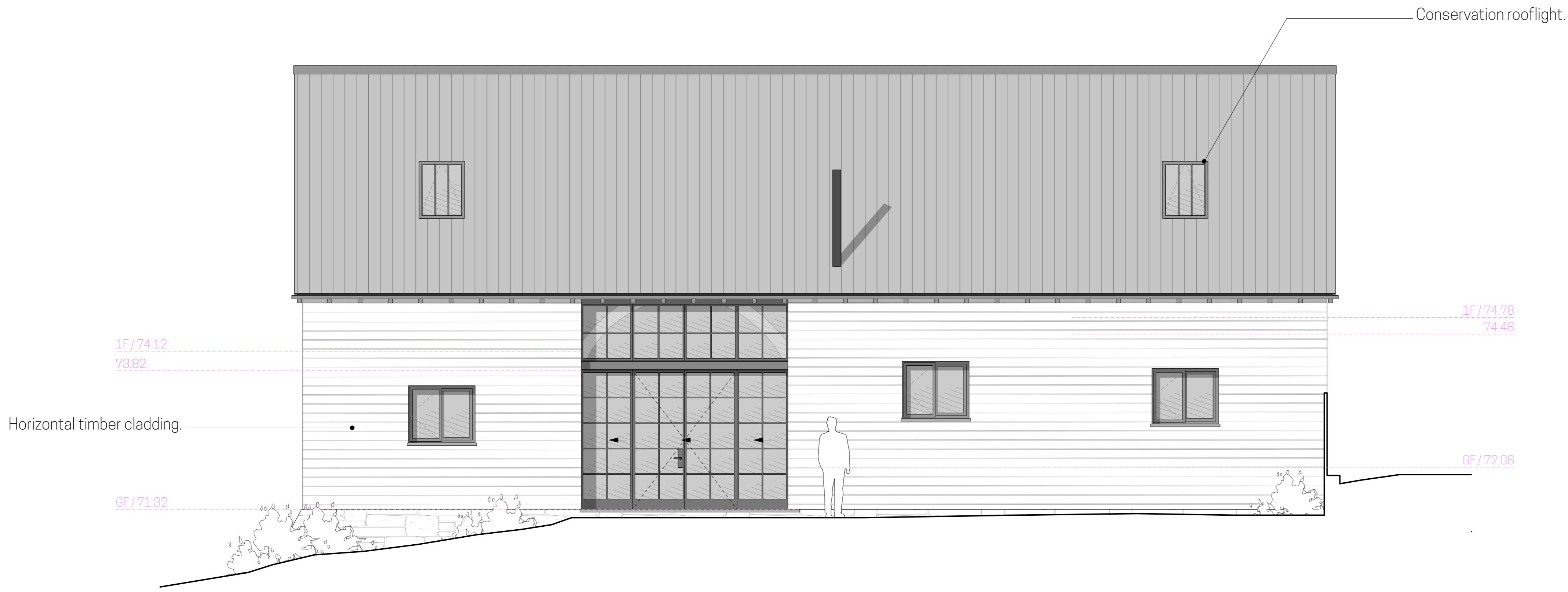
ELEVATION 03 [WEST] 1:50 @ A1 / 1:100 @ A3
