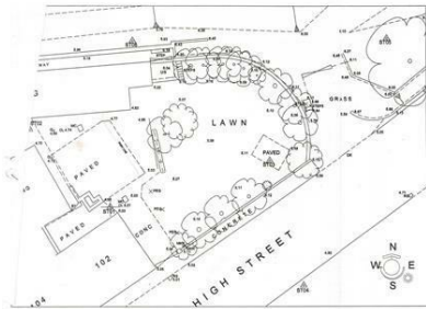
Site survey 1:200
