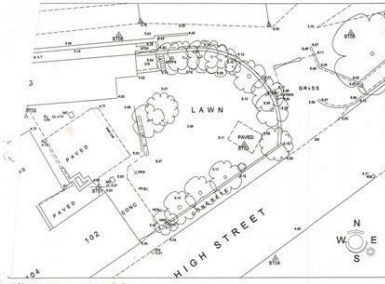
Site survey 1:200
