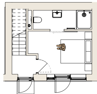
PLANS: G 1:50
