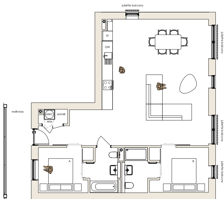
PLAN 1:50
