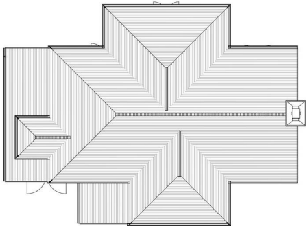
3 Roof Plan 1 : 100
