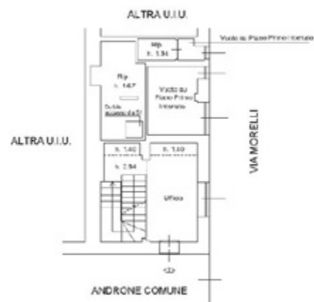
UFFICIO PIANO TERRA h. 5.20
