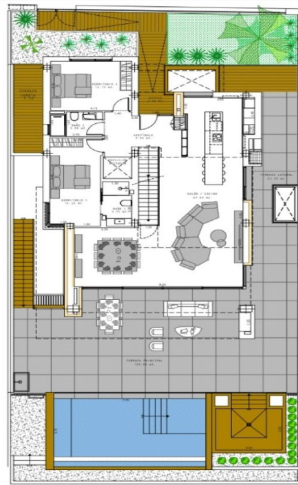
PLANTA BAJA
