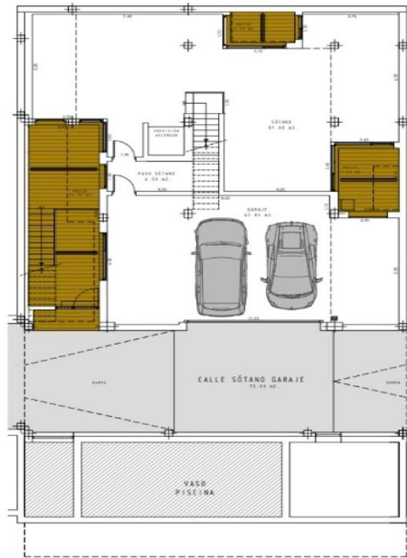
PLANTA SÓTANO
