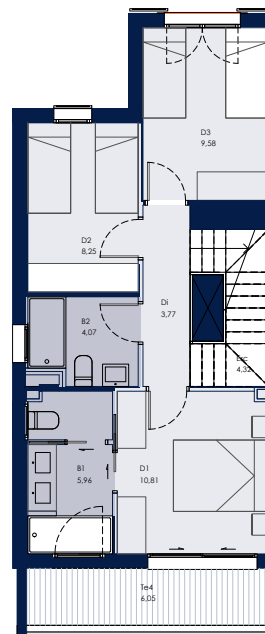
Planta Primera
