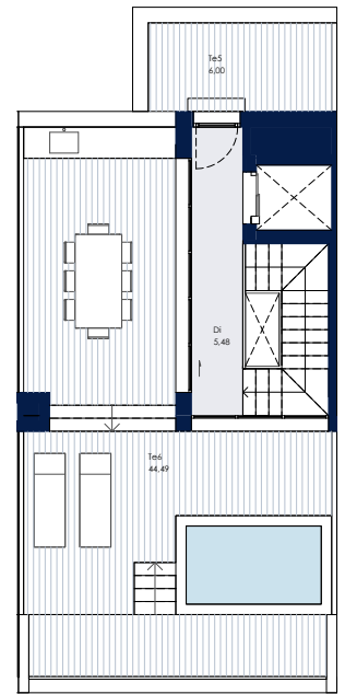
Planta Segunda
