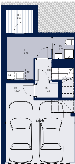
Planta Sótano
