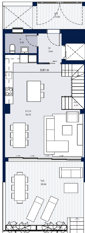
Planta Baja
