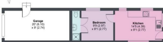
GARAGE / ANNEXE
