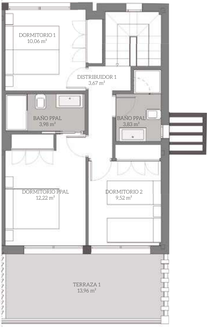
PLANTA ALTA
