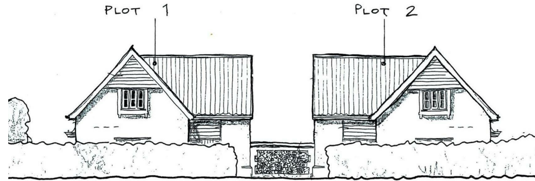
ELEVATION ~ 1:200
