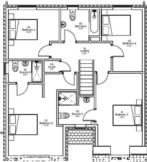
2 FF 1 : 50
