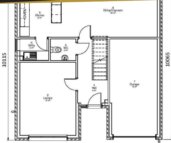
1 GF 1 : 50
