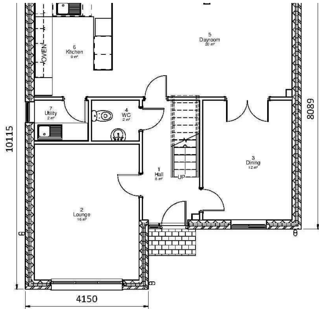
1 GF 1 : 50
