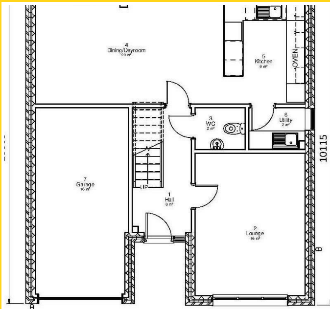
1 GF 1 : 50
